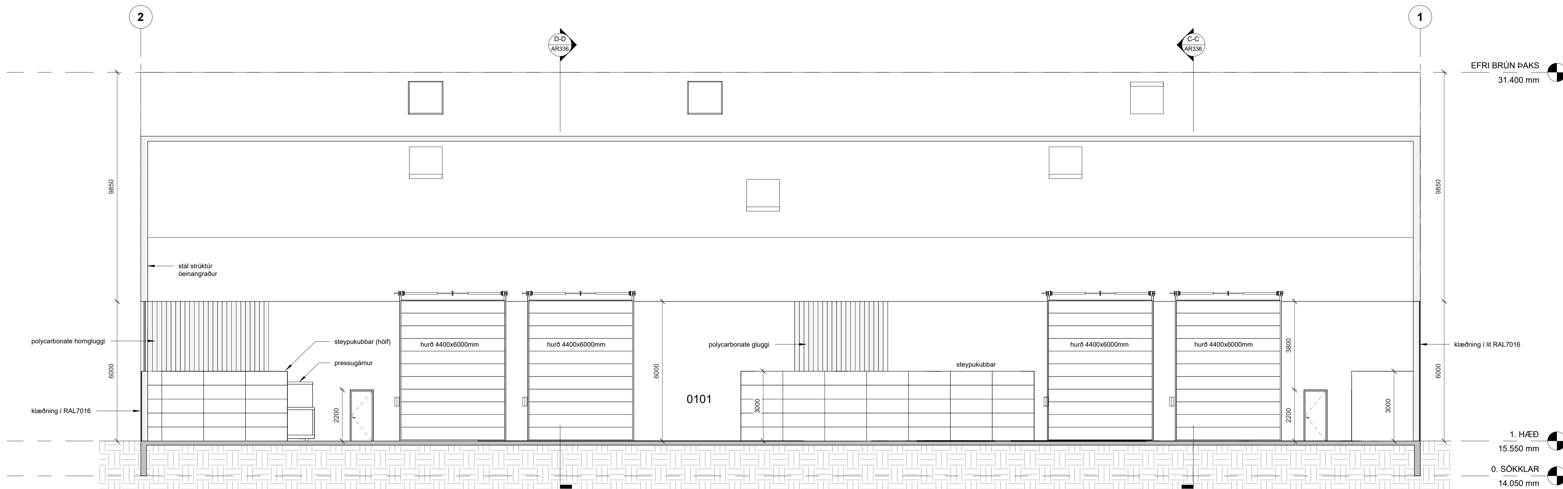
Snið A-A 1 : 100
